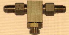
ラージ三方ニップルチーズ
